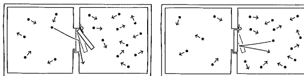
Fig. 6. Smoluchowski trapdoor.
